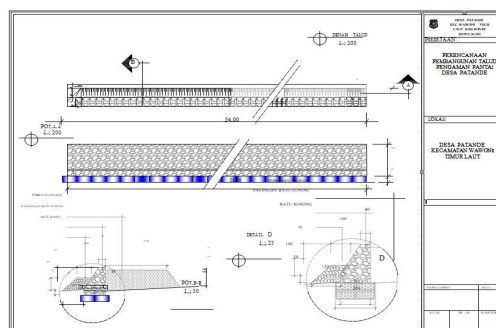
Gambar 4 Gambar Rencana Pembangunan Talud Pengaman Pantai Desa Patande
