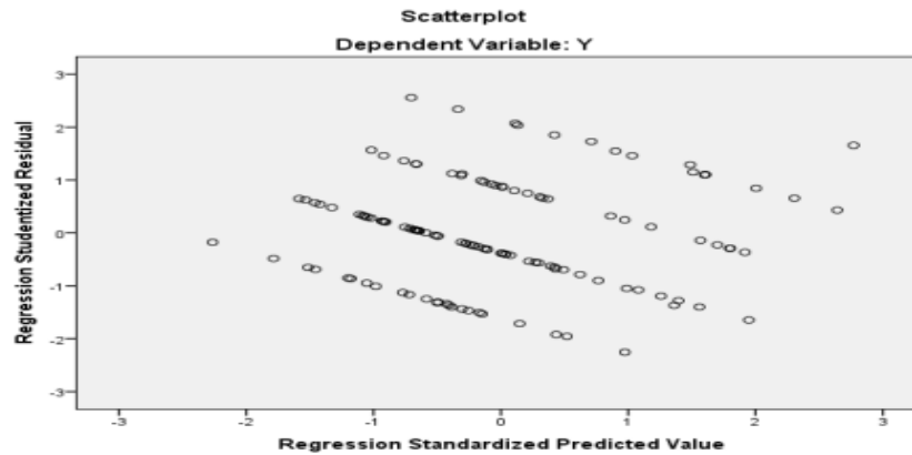
Gambar 2 Uji Heteroskedastitas
