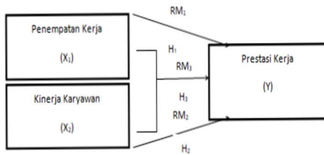
Gambar 1. Kerangka Berpikir
